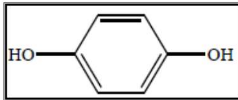
Gambar 1. Struktur Hidroquinone
